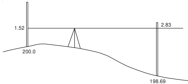
Fig. 8.2. Simple levelling
