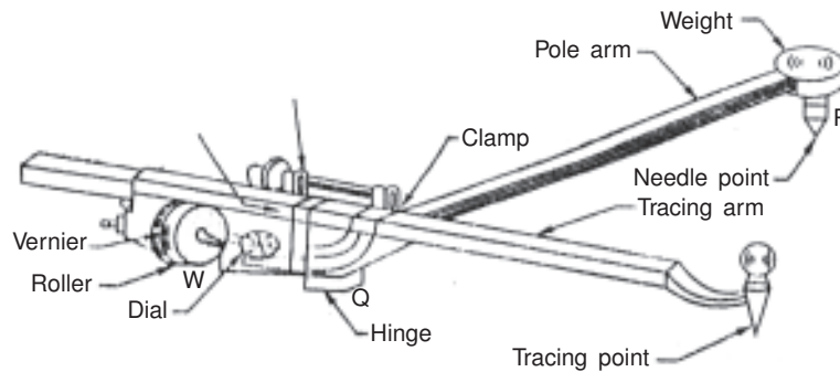
Fig. 7.6. Non-digital planimeter
