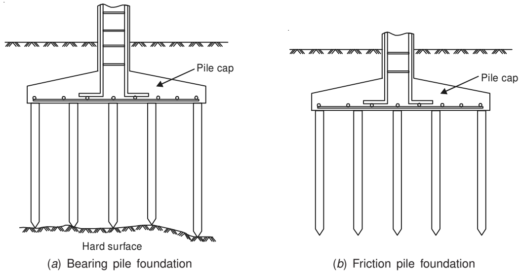
Fig. 4.9. Pile foundation
