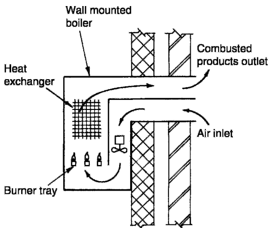
Fan at inlet
