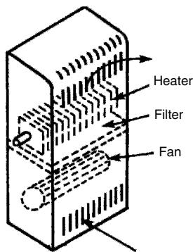
Fan convector
