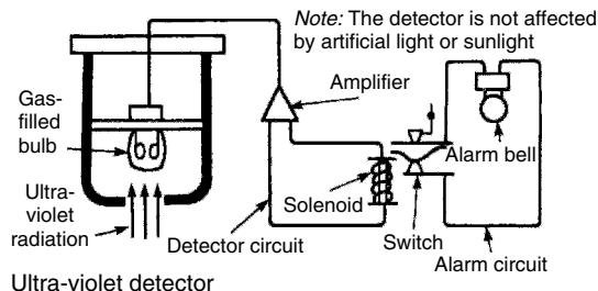
Ultra-violet detector
