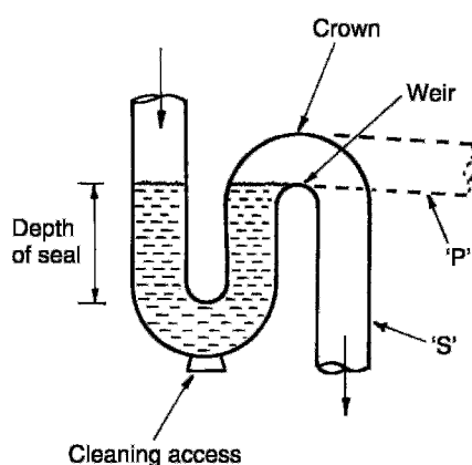
Tubular trap
