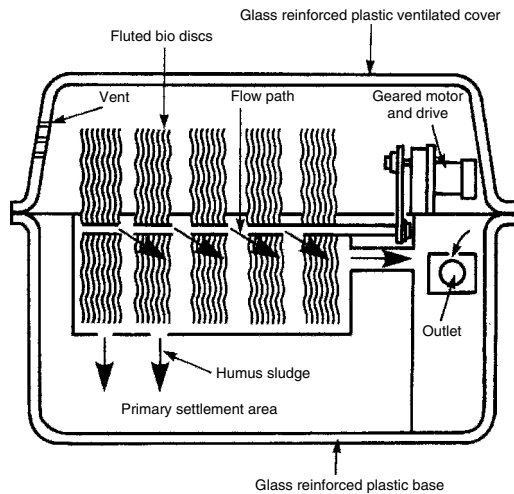
Longitudinal section
