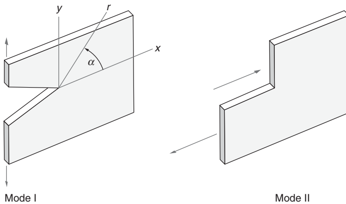
Figure 13-26 Coordinate system at the tip of the crack. (From Piltner, R., Spezielle finite element Lochen, Echen und Rissen, unter Verwendung von analytischen teillosunge , VDI-Verlag, Dusseldorf, No. 96, 1982).
